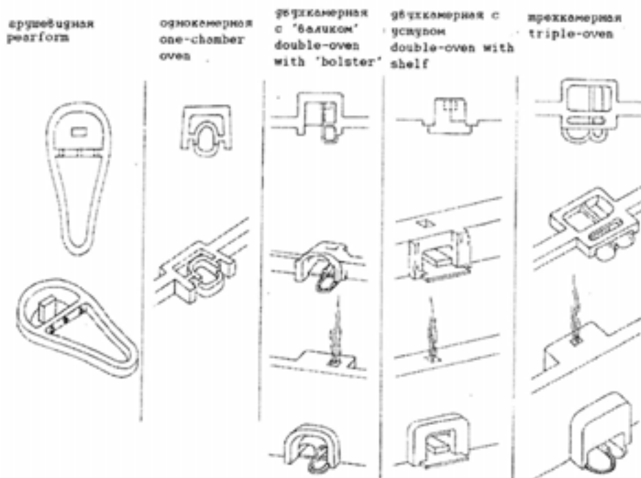
12. Demirgazyk Goňurdaky dini dâp-dessur äheňli ögjaklaryň görnüşleri Fig.12. Types of cult ovens of North Gonur Илл.12. Типы культовых печей Северного Гонура
