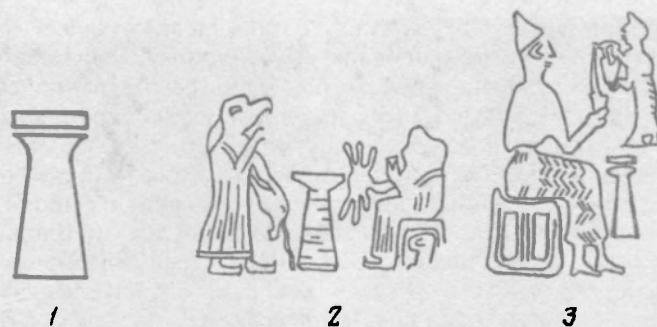
Рис. 7. «Миниатюрные колонки»: 1 — каменная «миниатюрная колонка» с крышкой из храма Тоголок-21; 2 — изображение «миниатюрной колонки» на хеттской печати; 3 — изображение «миниатюрной колонки» с крышкой на печати анатолийской группы
