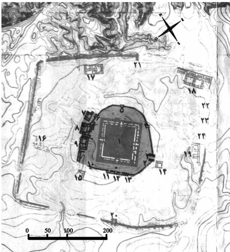
Схема центральной части зиккурата в Чога Занбиле (Иран). Shem of the central part of the Ziggurat in Choga-Zanbil (Iran)
